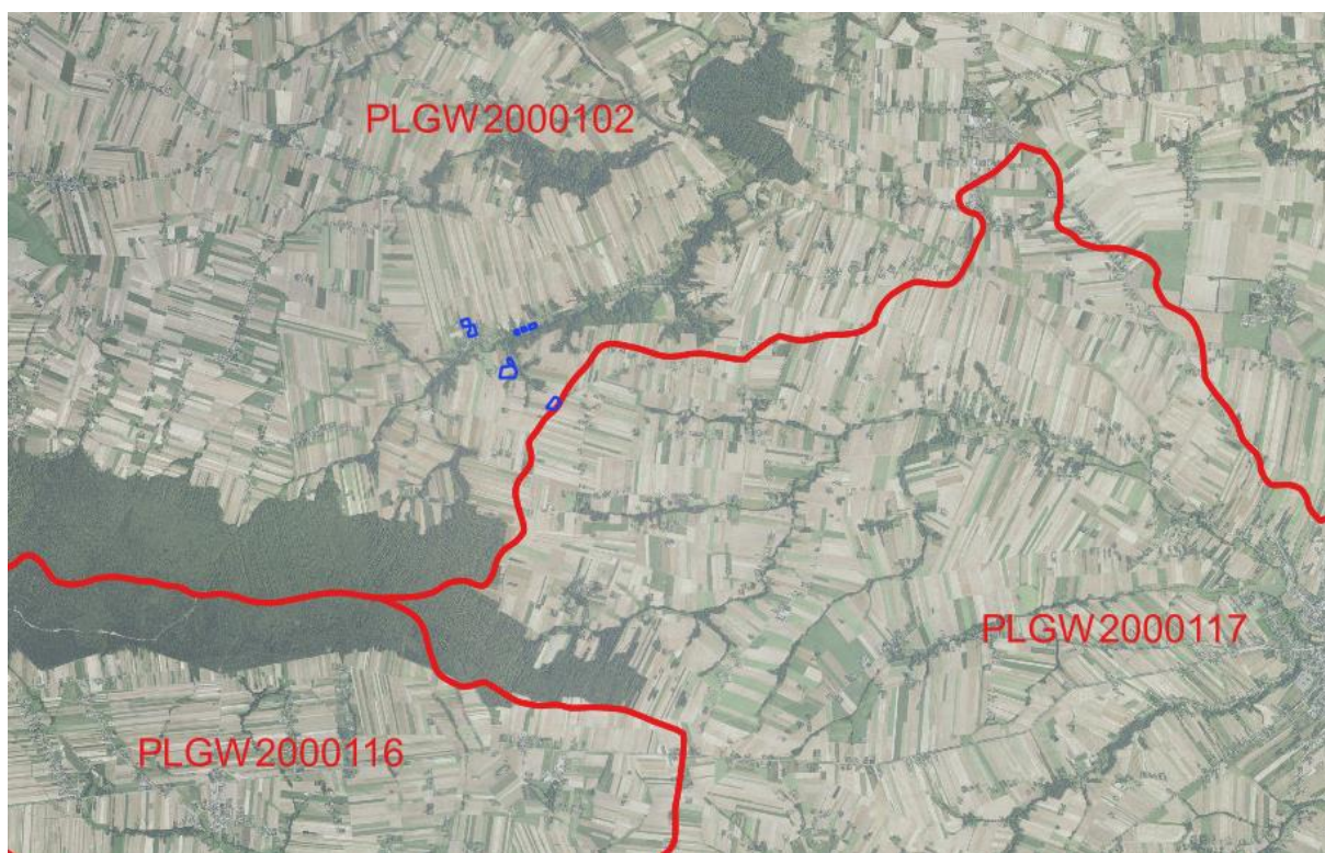
Rysunek 16. Granice JCWPd 102 w podziale na 172 jednostki (2009 r.) [źródło: Państwowa Służba Hydrogeologiczna]
